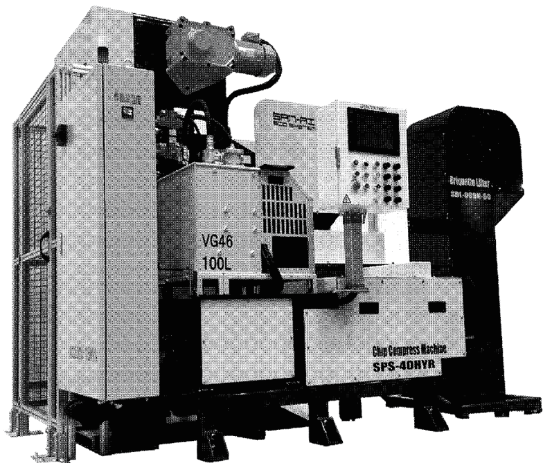
切粉圧縮機(付帯装置複合例)
